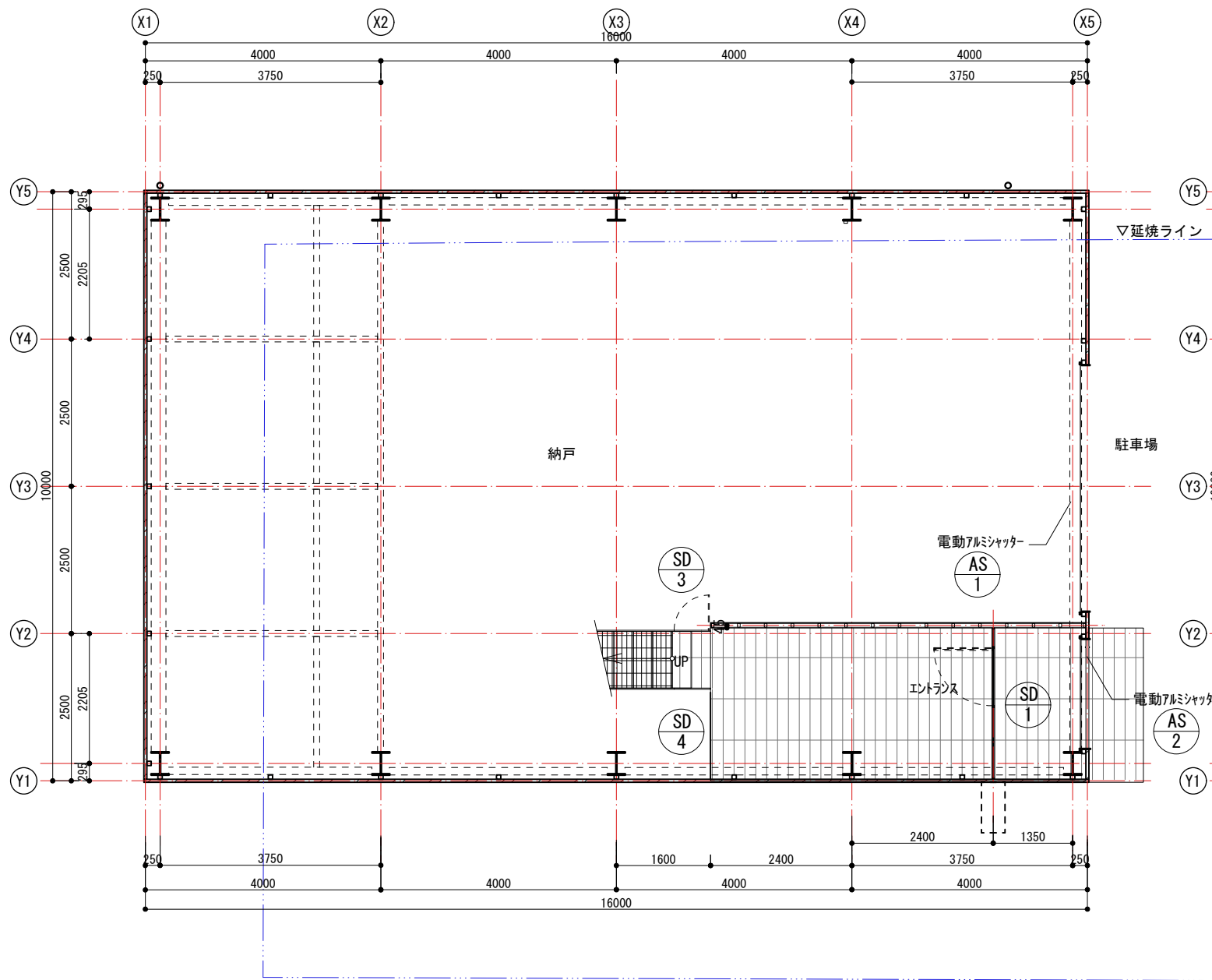
1階平面図
